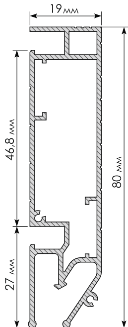
Профиль ЛБ 80 от Prozet
